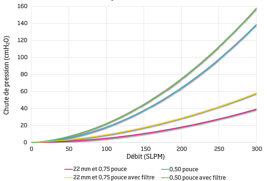
Chute de pression du 5300 Series
